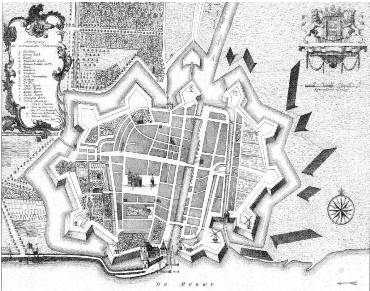
Grondtekening van de stad Gorinchem uit 1755 met onder meer het Pesthuis, De Tol en een "Nieuw Magazijn": het Arsenal.
