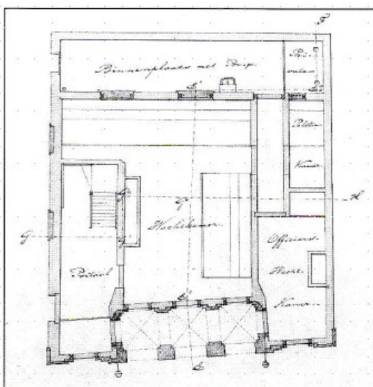
De begane grond van de Hoofdwacht met een wachtkamer voor 20 à 25 soldaten en een wachtkamer voor officieren. De politiekamer diende als arrestantenlokaal (foto van het Algemeen Rijksarchief van een tekening uit 1854 door ingenieur J. Carsten).
